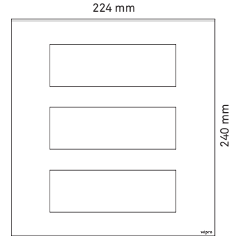
18 Module Plate
