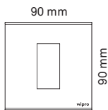
1 Module Plate
